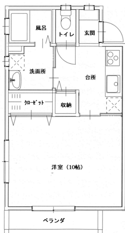
図 1.参考間取図
