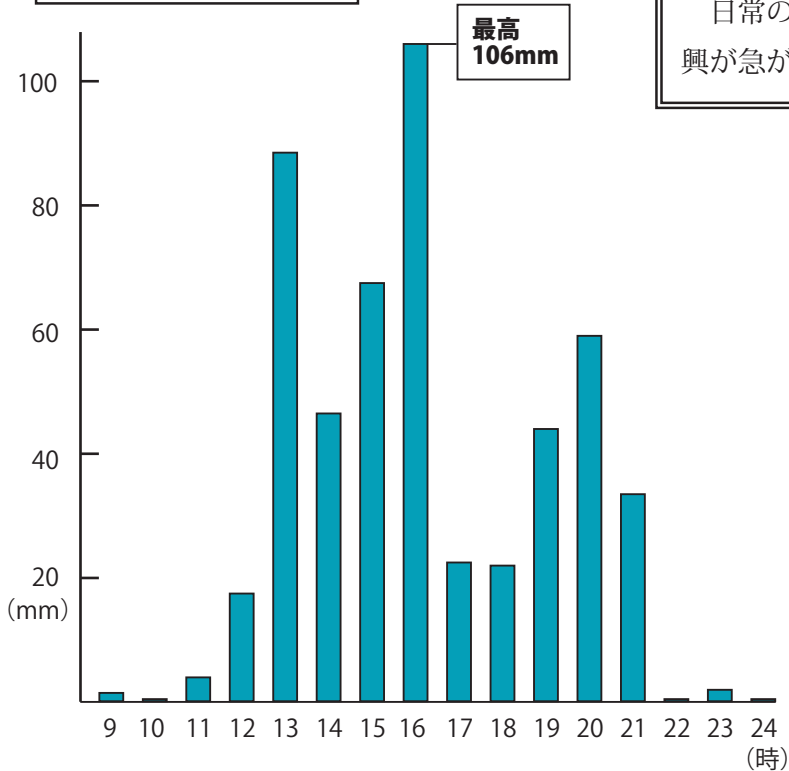
5日の雨量グラフ
